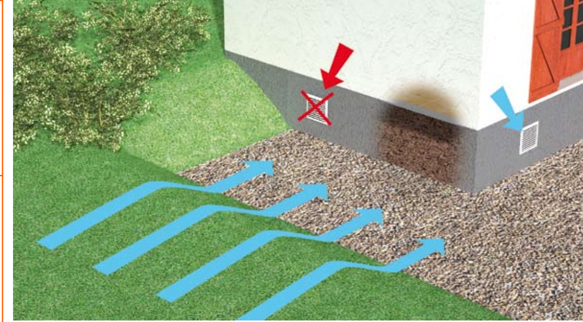
Disposition des grilles de ventilation du vide sanitaire par rapport au sens du courant
