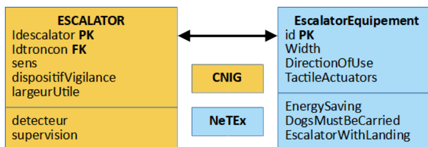
Schéma 06 - Escalator
