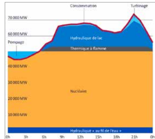
Production électrique schématisée d'une journée d'hiver en France © DR
