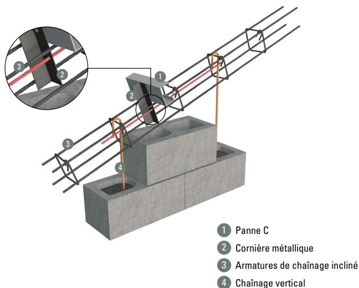
Figure 19 : Jonction panne de charpente sur chaînage incliné
