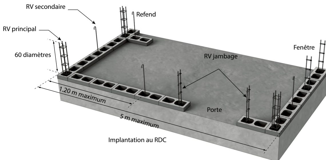
Figure 15 : Exemple de chaînages verticaux
