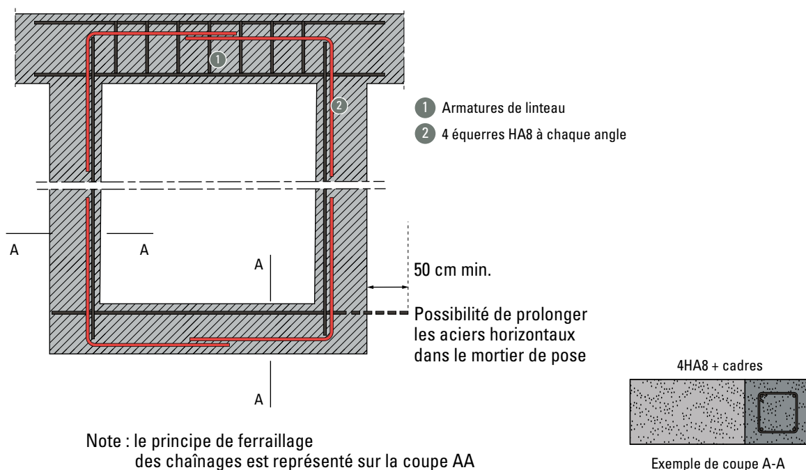
Figure 17 : Disposition des armatures des ouvertures et des baies
