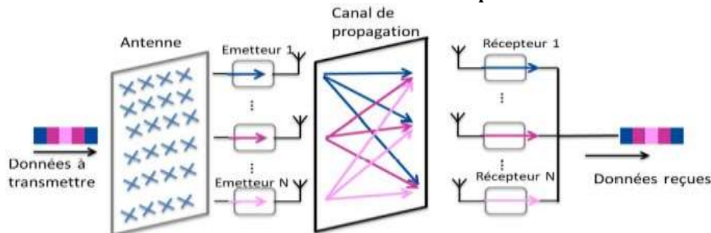
Illustration 2 : Illustration de la technique « MIMO »
