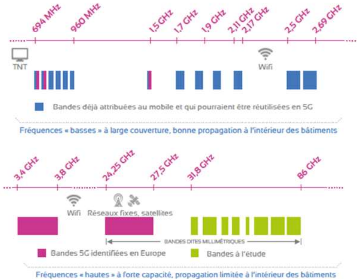
Graphique 2 : Fréquences utilisées pour la 5G
