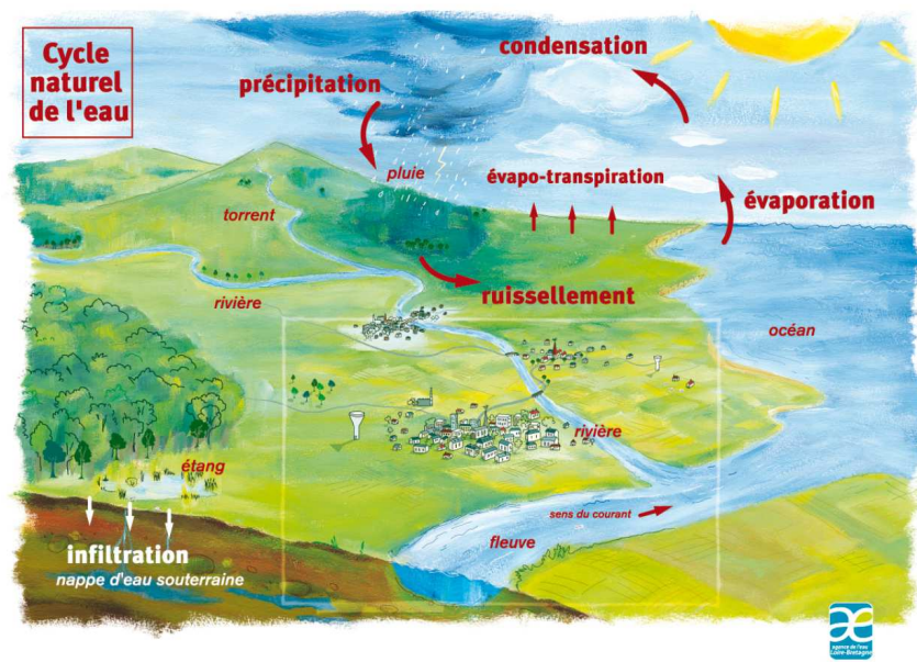
Illustration 3 : le grand cycle de l'eau (Agence de l'eau Loire Bretagne)
