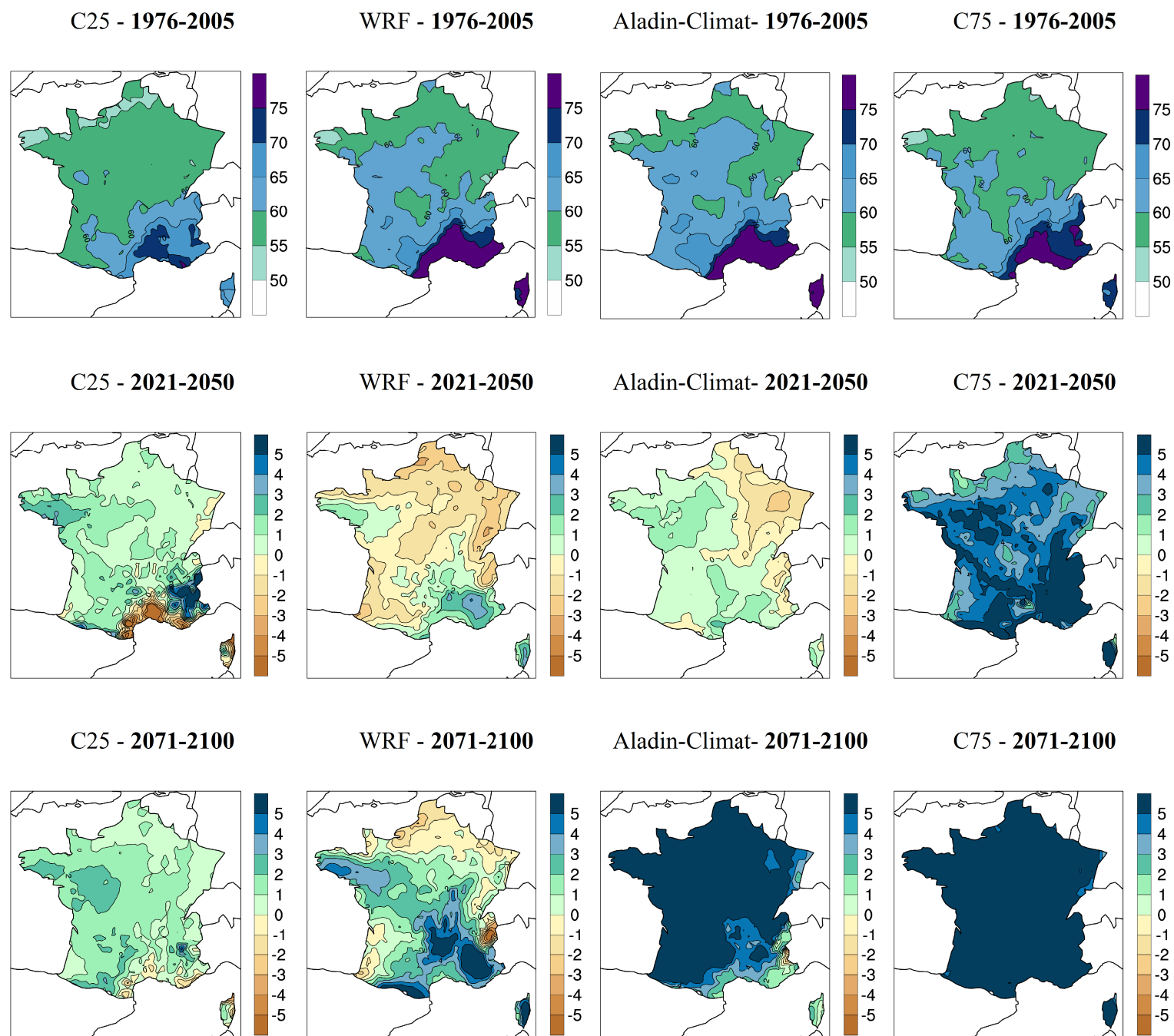
Figure 18: Pourcentage des précipitations extrêmes annuelles, pour la période de référence 1976-2005 (ligne du haut) et les écarts à cette référence pour le scénario RCP8.5 , aux horizons 2021-2050 (ligne du milieu) et 2071-2100 (ligne du bas). Pour chaque ligne, de gauche à droite : 25 e centile de l'ensemble, WRF, Aladin-Climat, 75 e centile de l'ensemble.
