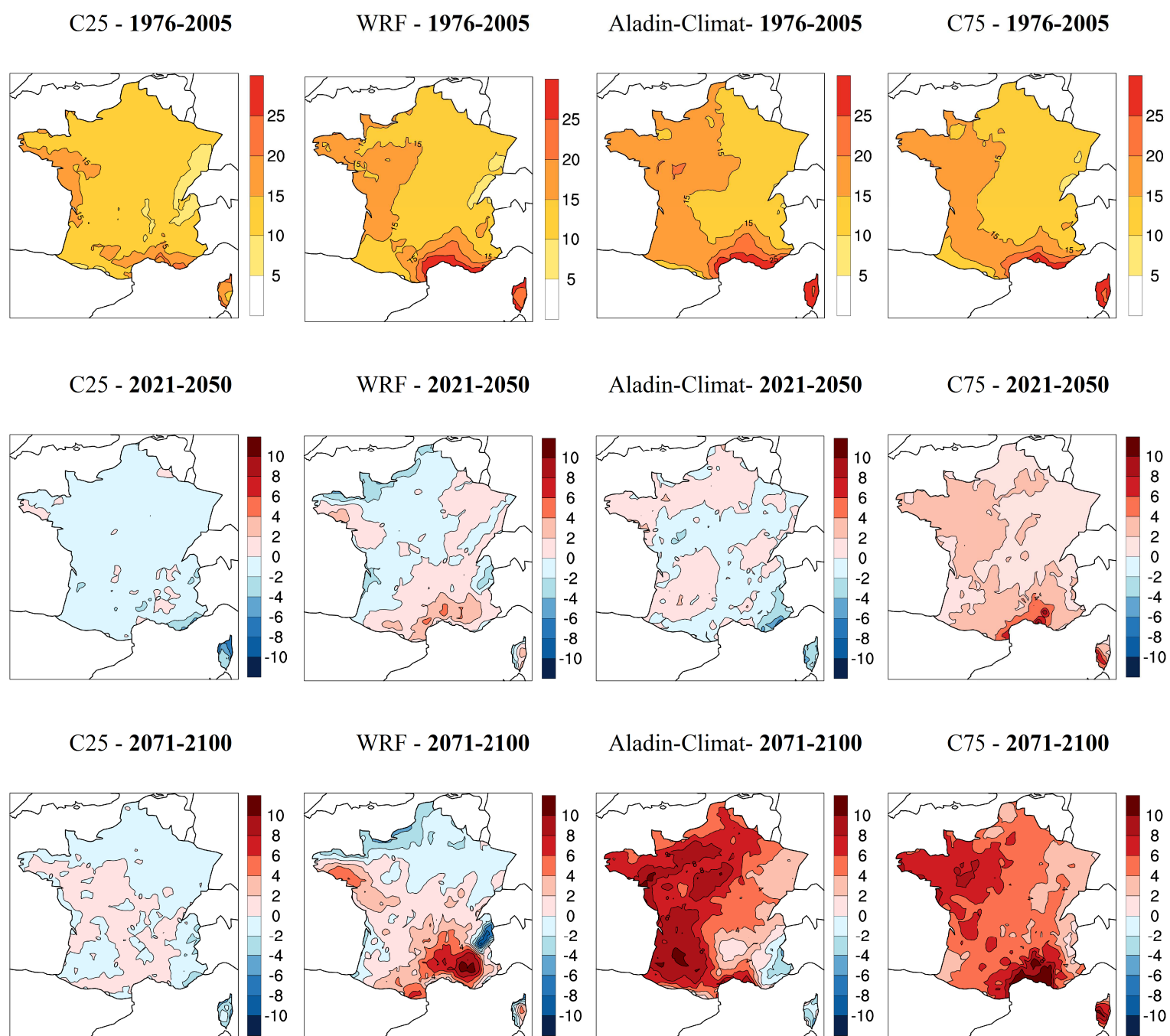
Figure 20: Nombre de jours consécutifs avec moins de 1 mm de précipitations estivales, pour la période de référence 1976-2005 (ligne du haut) et les écarts à cette référence pour le scénario RCP8.5 , aux horizons 2021-2050 (ligne du milieu) et 2071-2100 (ligne du bas). Pour chaque ligne, de gauche à droite : 25 e centile de l'ensemble, WRF, Aladin-Climat, 75 e centile de l'ensemble.
