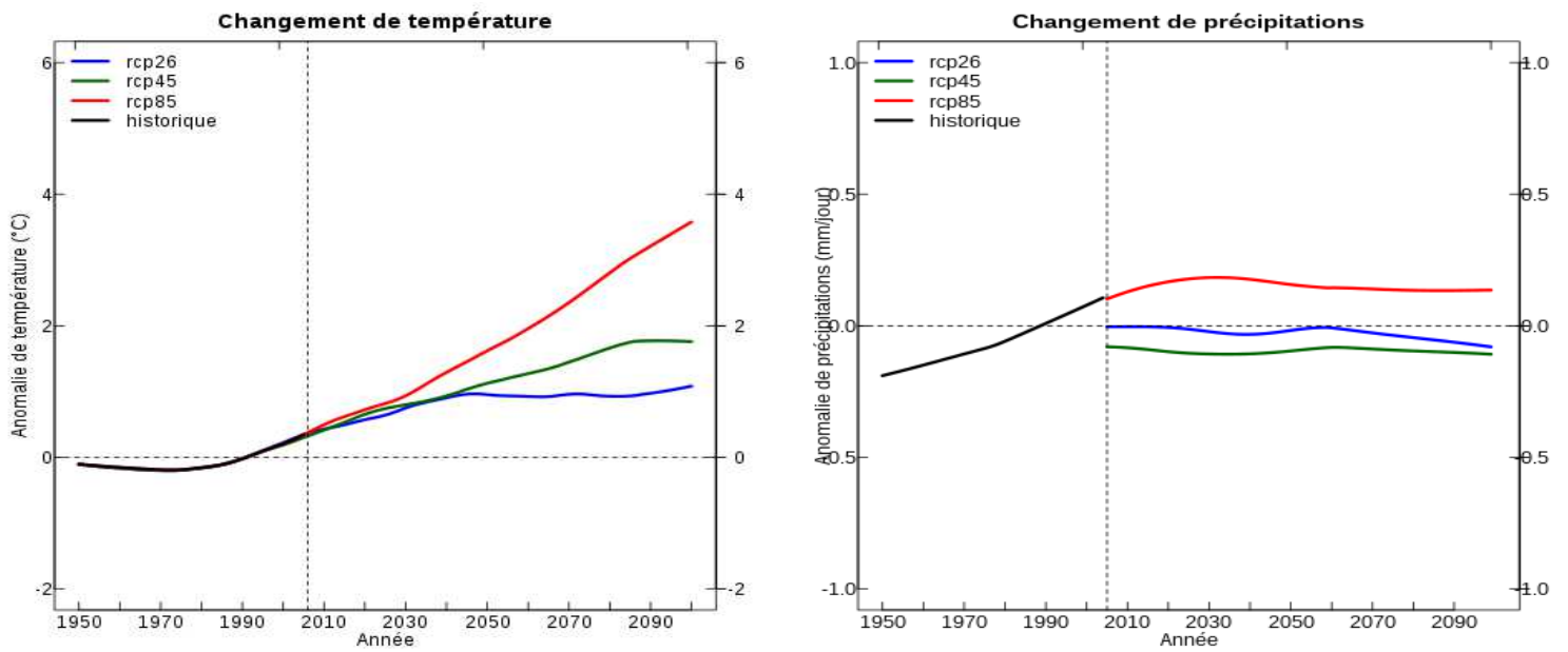
Figure 21: Evolution de la température (à gauche, en °C) et des précipitations (à droite, en mm/jour), relativement à la référence 1976-2005, pour les scénarios RCP2.6 en bleu, RCP4.5 en vert et RCP8.5 en rouge.
