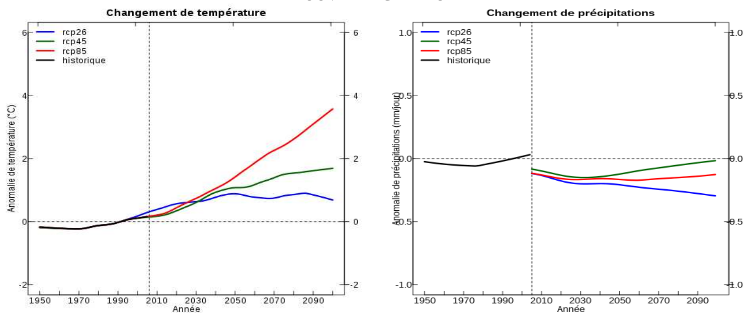
Figure 22: Evolution de la température (à gauche, en °C) et des précipitations (à droite, en mm/jour), relativement à la climatologie 1976-2005, pour les scénarios RCP2.6 en bleu, RCP4.5 en vert et RCP8.5 en rouge.
