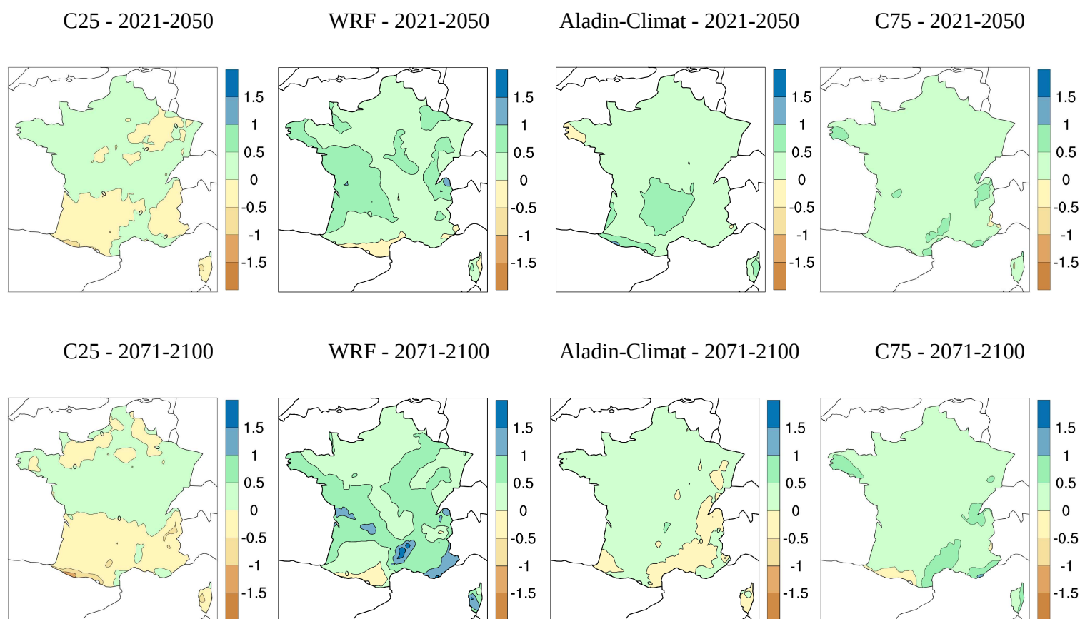
Figure 9: Écarts de précipitations hivernales (mm/jour) en France relative à la référence 1976-2005, pour le scénario RCP4.5, aux horizons 2021-2050 et 2071-2100. Pour chaque ligne, de gauche à droite : 25 e centile de l'ensemble, WRF, Aladin-Climat, 75 e centile de l'ensemble.
