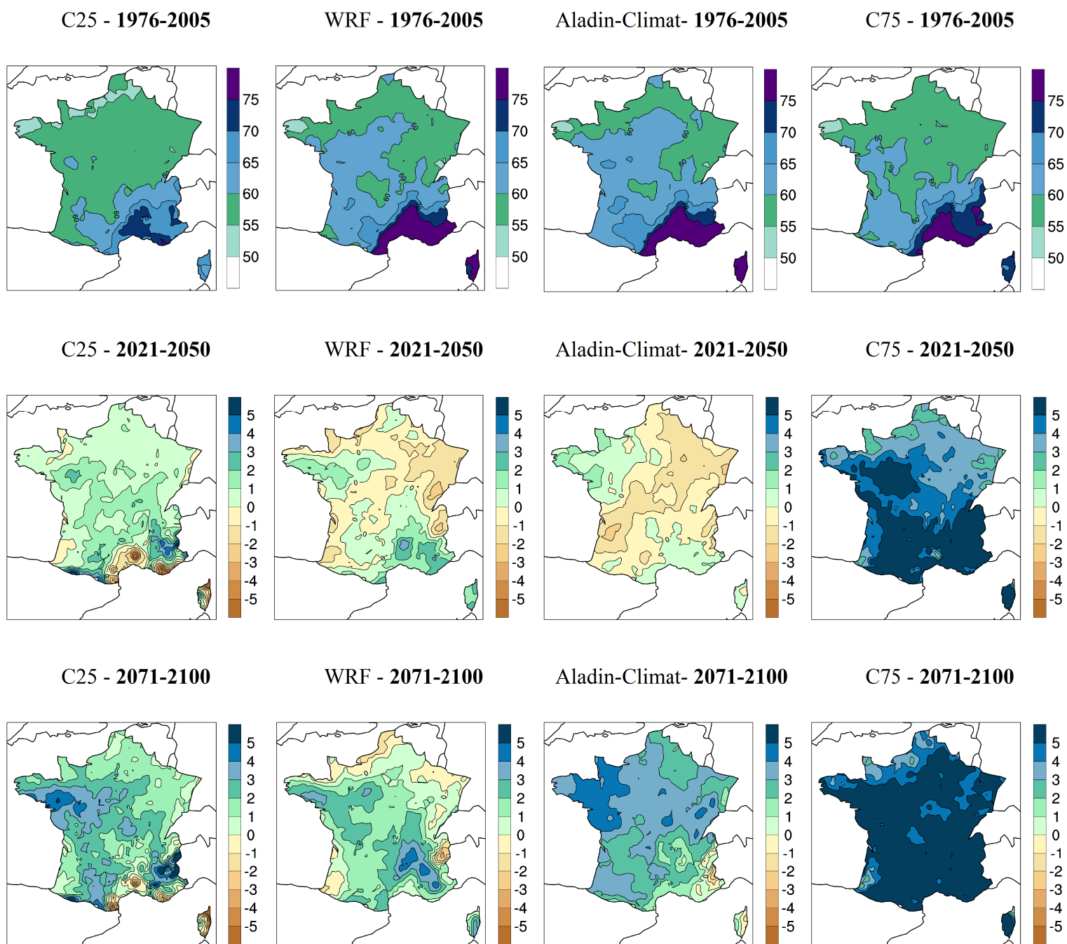
Figure 17: Pourcentage des précipitations extrêmes annuelles, pour la période de référence 1976-2005 (ligne du haut) et les écarts à cette référence pour le scénario RCP4.5 , aux horizons 2021-2050 (ligne du milieu) et 2071-2100 (ligne du bas). Pour chaque ligne, de gauche à droite : 25 e centile de l'ensemble, WRF, Aladin-Climat, 75 e centile de l'ensemble.
