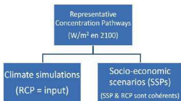
Figure 1 : Élaboration en parallèle des scénarios climatiques et socio-économiques (d'après Noorwijkhout).
