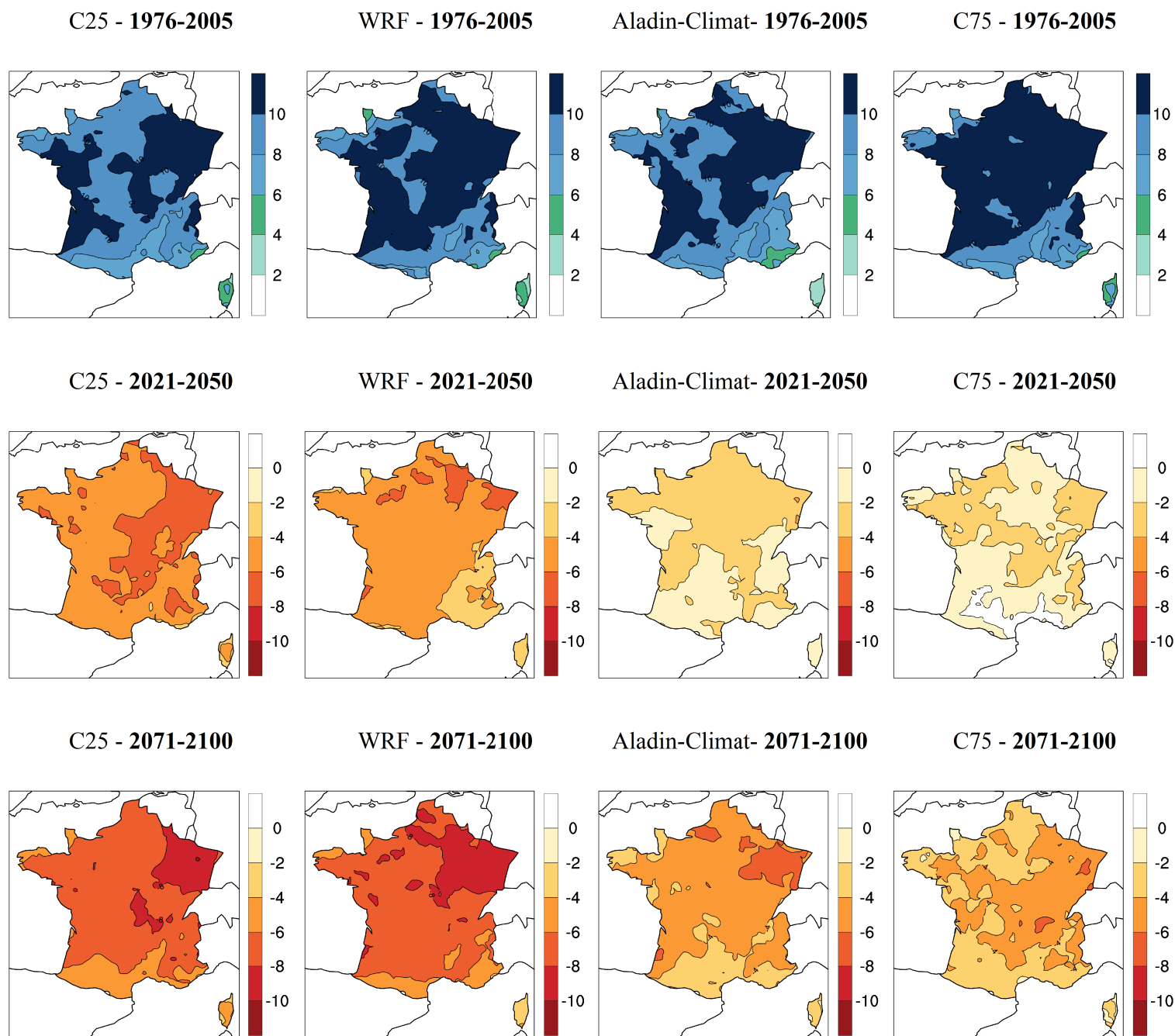
Figure 15: Nombre de jours hivernaux à température anormalement basse, pour la période de référence 1976-2005 (ligne du haut) et les écarts à cette référence pour le scénario RCP4.5 , aux horizons 2021-2050 (ligne du milieu) et 2071-2100 (ligne du bas). Pour chaque ligne, de gauche à droite : 25 e centile de l'ensemble, WRF, Aladin-Climat, 75 e centile de l'ensemble.
