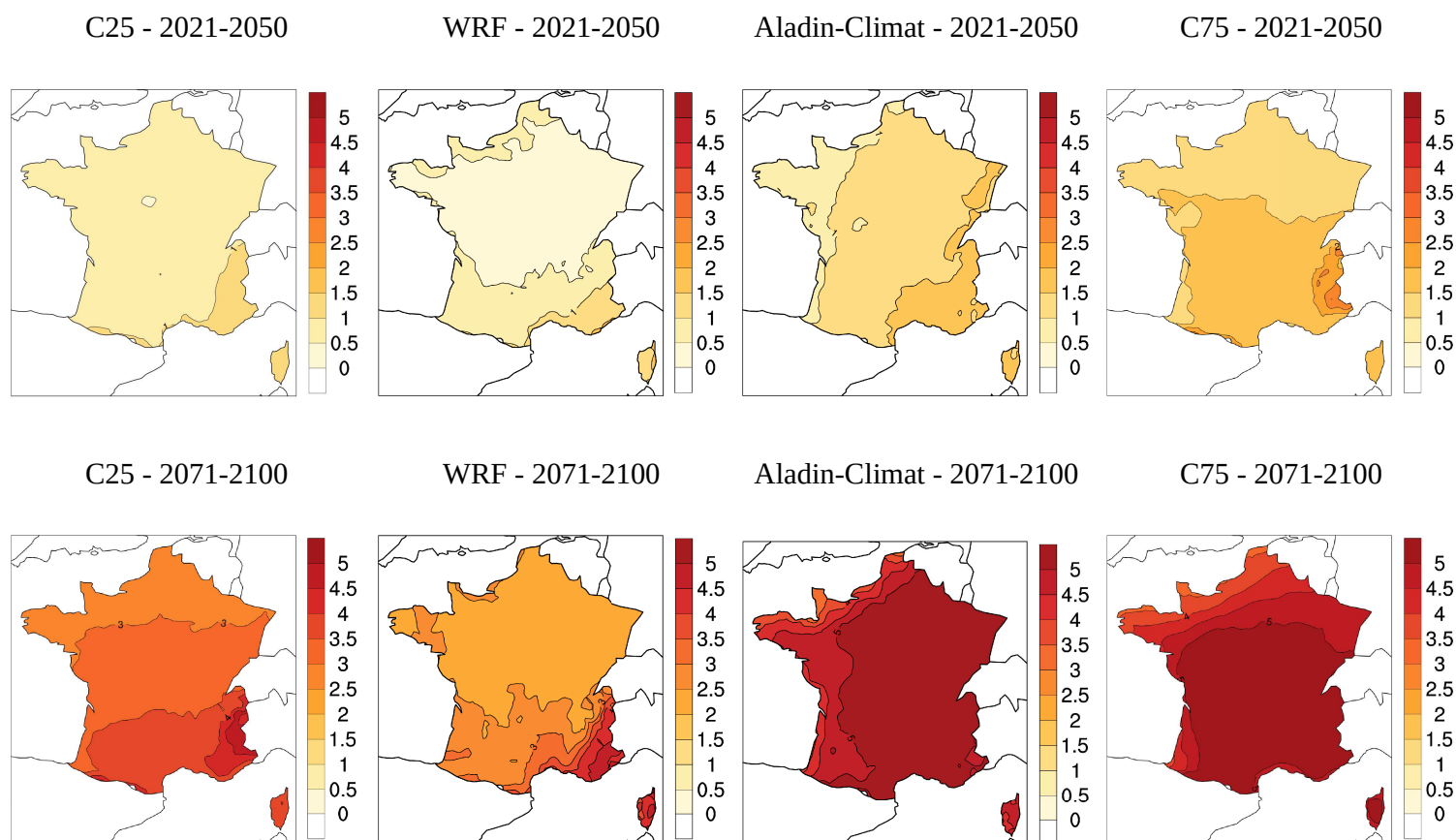
Figure 7: Écart de température estivale (°C) en France relativement à la référence 1976-2005, pour le scénario RCP8.5, aux horizons 2021-2050 et 2071-2100. Pour chaque ligne, de gauche à droite : 25 e centile de l'ensemble, WRF, Aladin-Climat, 75 e centile de l'ensemble.
