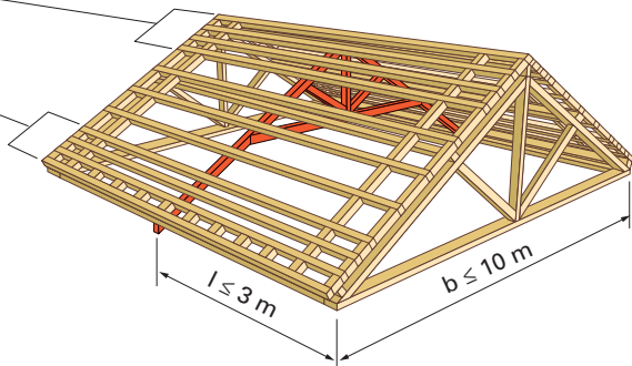
Figure 18 : Espacement des 4 premières pannes d'extrémité
