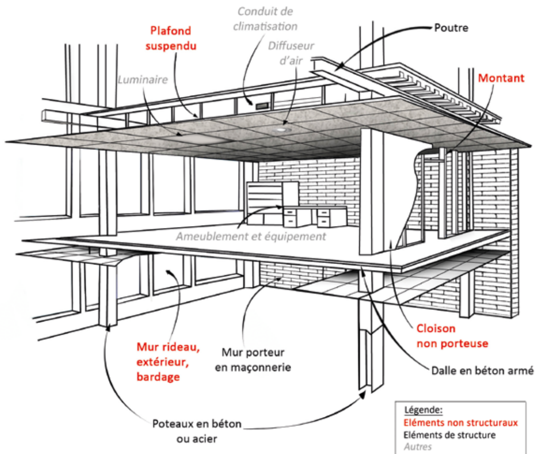
Figure 1-1 : Distinction de certains éléments non structuraux du cadre bâti
