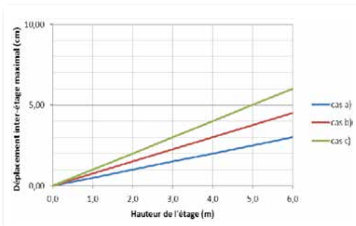
Figure 2-4: Valeurs des déplacements inter-étages maximaux sous séisme fréquent pour un bâtiment neuf
