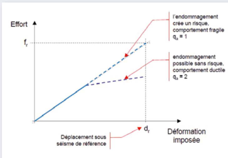
Figure 2-1 : Principe du coefficient de comportement q_a
