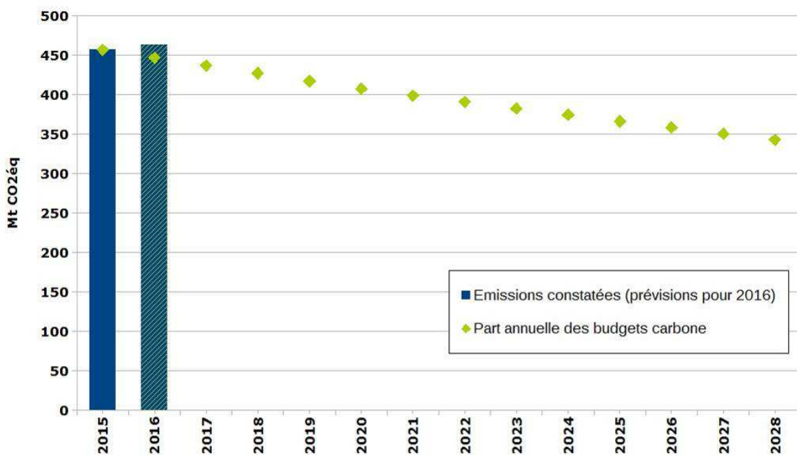
Evolution des émissions de gaz à effet de serre du secteur "transports" en France et objectifs SNBC (parts sectorielles des budgets-carbone 2015-2018, 2019-2023 et 2024-2028)
