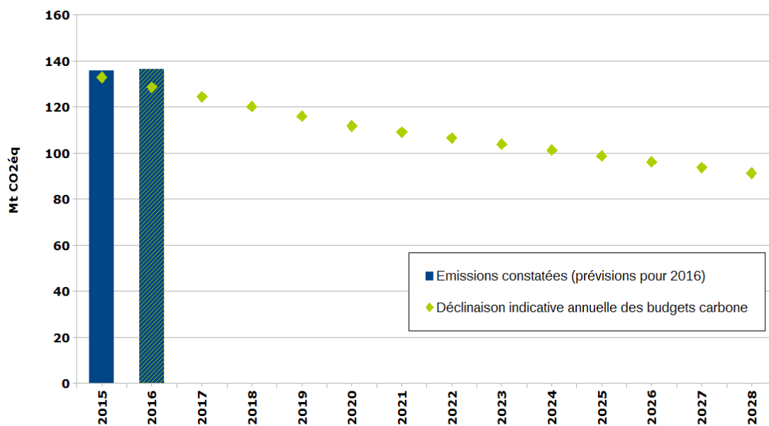
Evolution des émissions de gaz à effet de serre du secteur "transports" en France et objectifs SNBC (parts sectorielles des budgets-carbone 2015-2018, 2019-2023 et 2024-2028)
